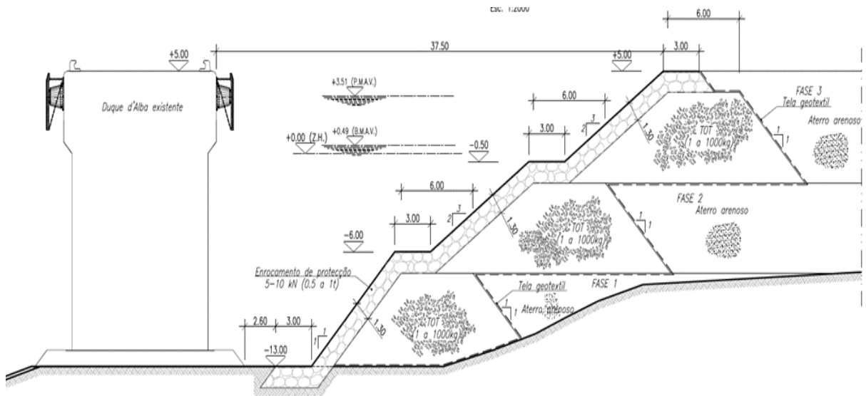
Figura 3.1 - Corte elucidativo da solução proposta para de contenção do aterro na zona nascente do terminal Ro-ro
